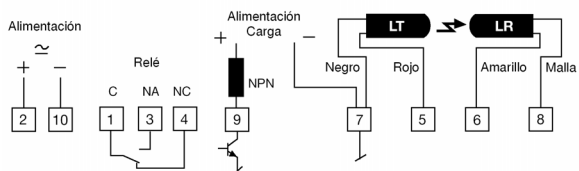
Salida Relé/Transistor – PA 11 A/B 30XT
