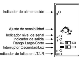
PA 11 B xxx
