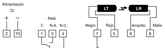
Salida relé – PA 10 A/B 51X
