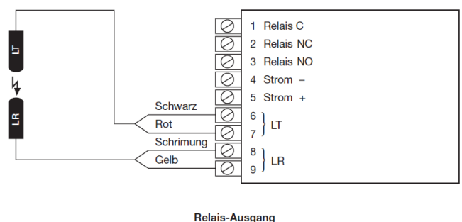
Relais-Ausgang
