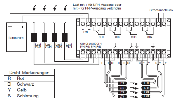
MPA 41 A/C
